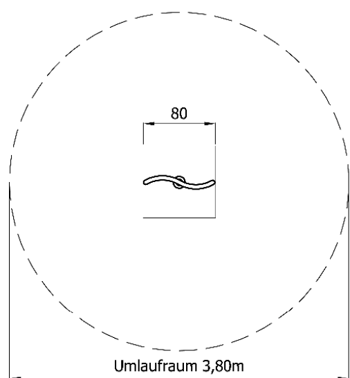
11 3311 drehbar/gewellt
