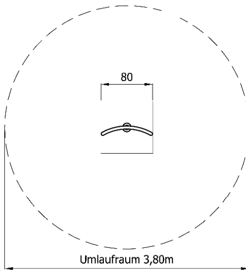
11 3310 drehbar/gebogen
